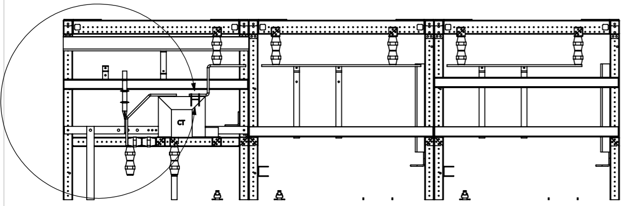
SECTION G-G SCALE 1 : 20
